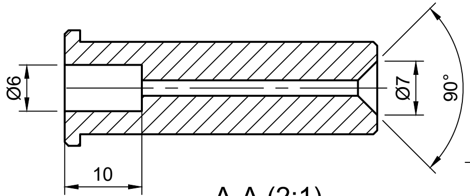
A-A (2:1)
