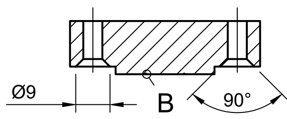
A-A (1:1)
